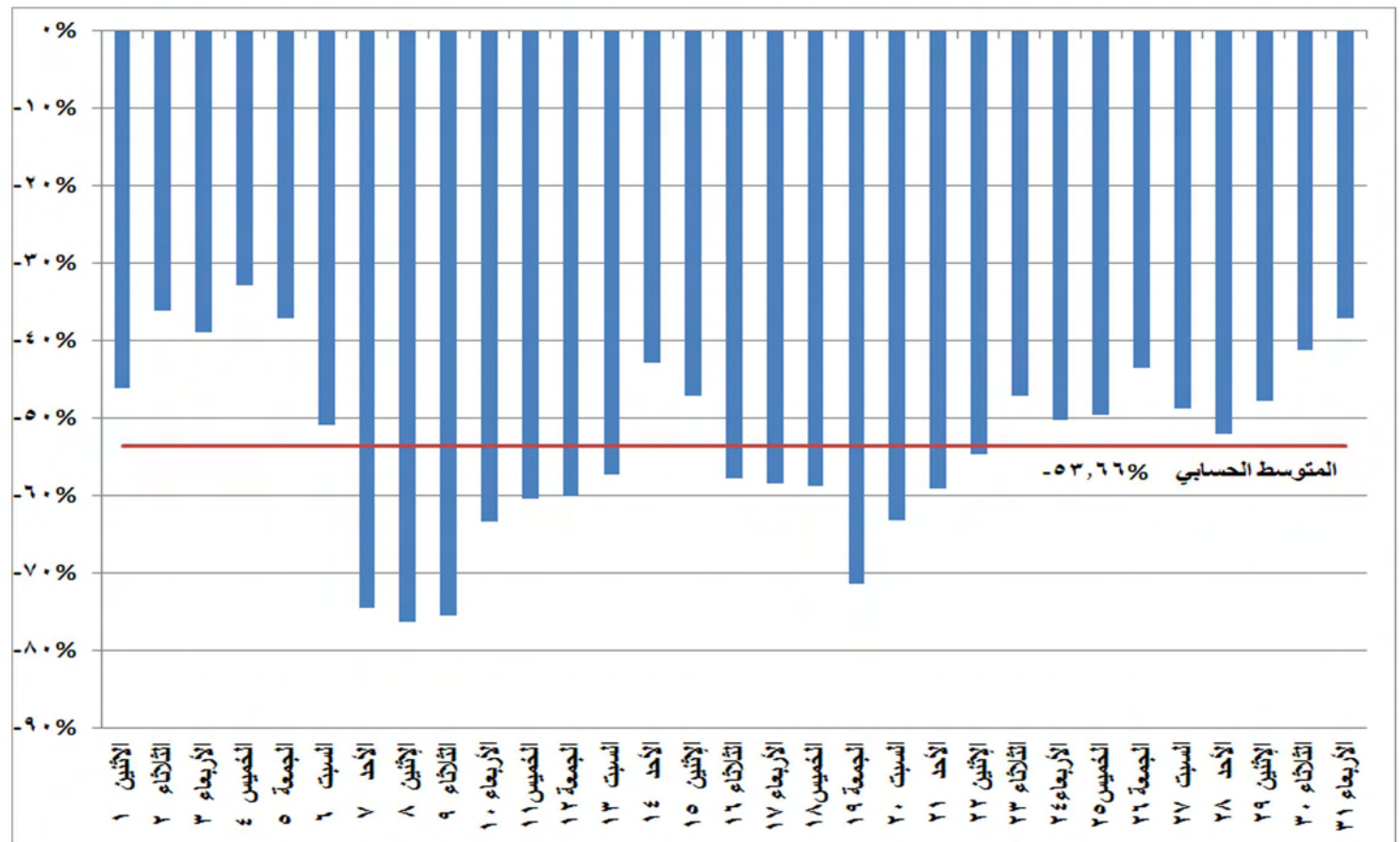
شكل (٢٠) نسب التغير في استخدام المازوت في إنتاج الطاقة الكهربائية خلال شهر أكتوبر ٢٠١٨ مقارنة بالشهر المماثل من العام السابق
