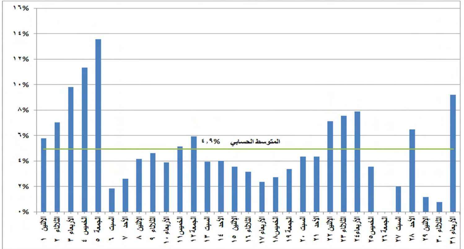
شكل (٩) النسب المئوية للتغير في الحمل الاقصى خلال شهر أكتوبر ٢٠١٨ مقارنة باليوم المماثل من العام الماضي
