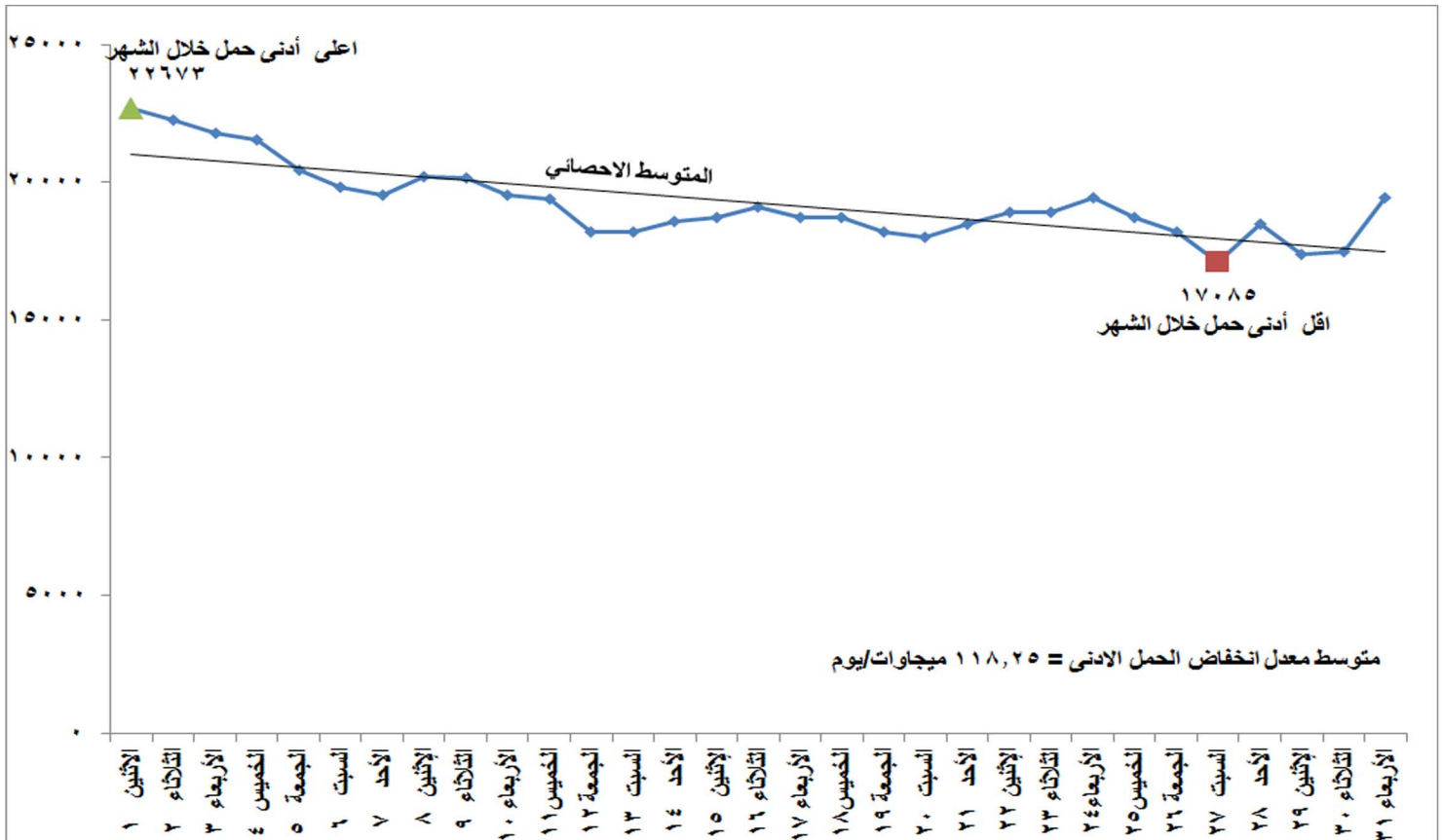
شكل (٢) تطور الحمل الادنى اليومي خلال شهر أكتوبر ٢٠١٨
