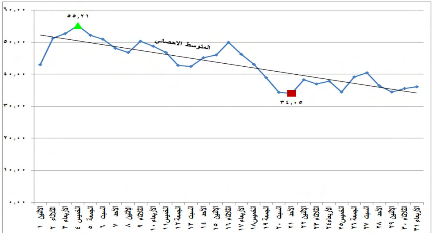
شكل (٢١) الطاقة الكهربائية المنتجة من المصادر غير الحرارية خلال شهر أكتوبر ٢٠١٨
