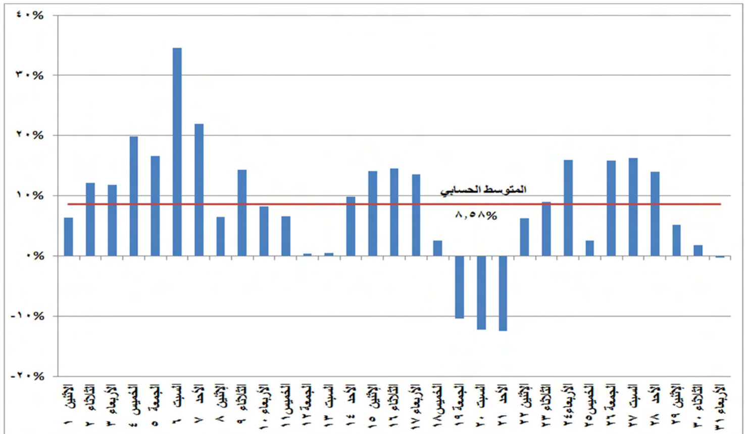
شكل (٢٢) نسب التغير في استخدام المصادر غير الحرارية في إنتاج الطاقة الكهربائية خلال شهر أكتوبر ٢٠١٨ مقارنة بالشهر المماثل من العام السابق
