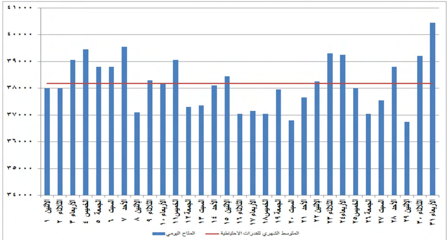
شكل (٢٧) القدرات المتاحة يوميا والمتوسط الشهري للقدرة الاحتياطية خلال شهر أكتوبر ٢٠١٨
