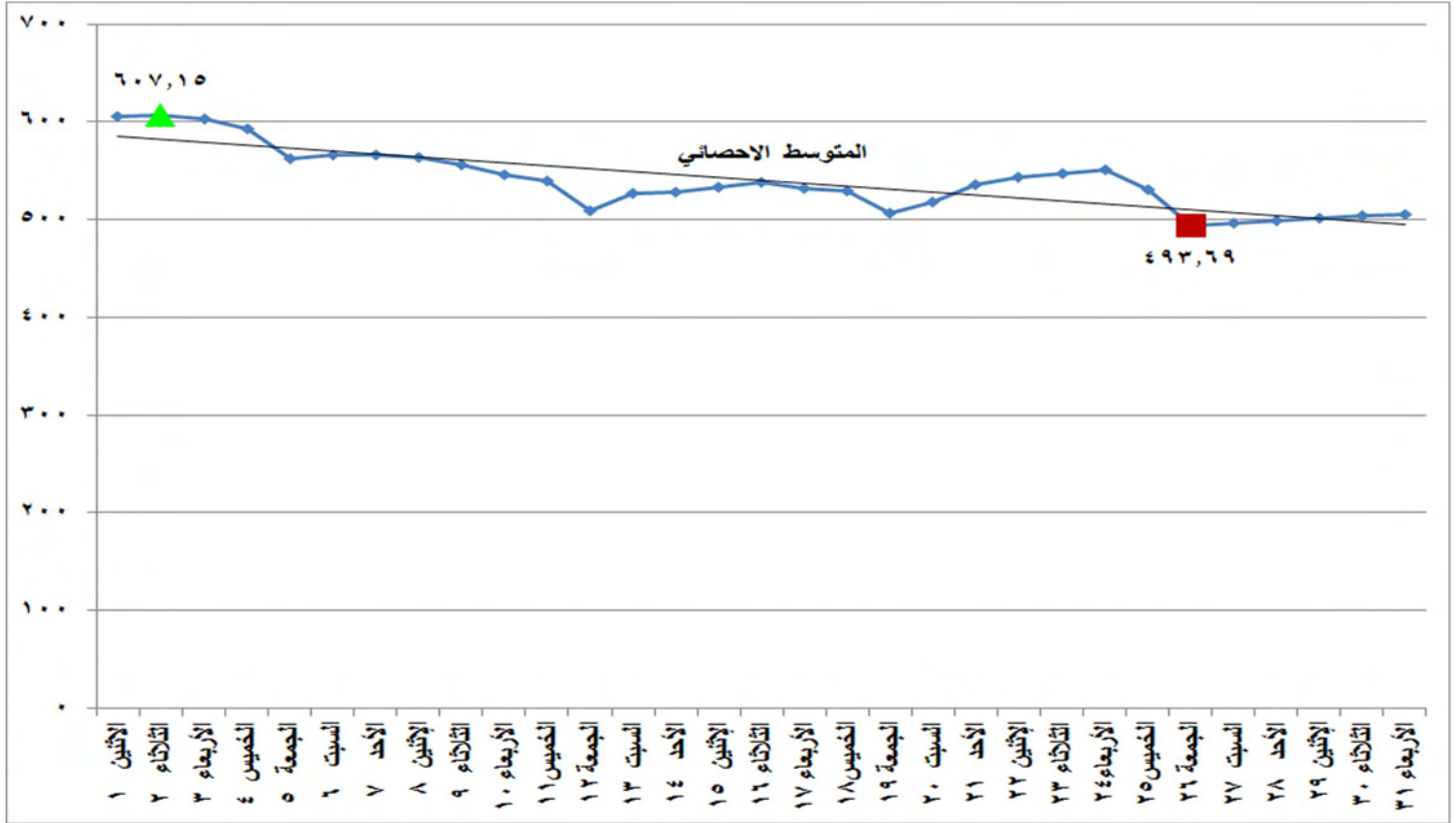
شكل (١٥) إجمالي الطاقة الكهربائية المنتجة من كل المصادر الأولية خلال شهر أكتوبر ٢٠١٨
