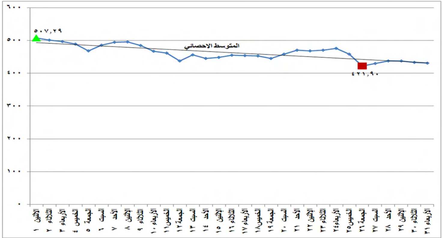
شكل (١٧) الطاقة الكهربائية المنتجة من الغاز الطبيعي خلال شهر أكتوبر ٢٠١٨
