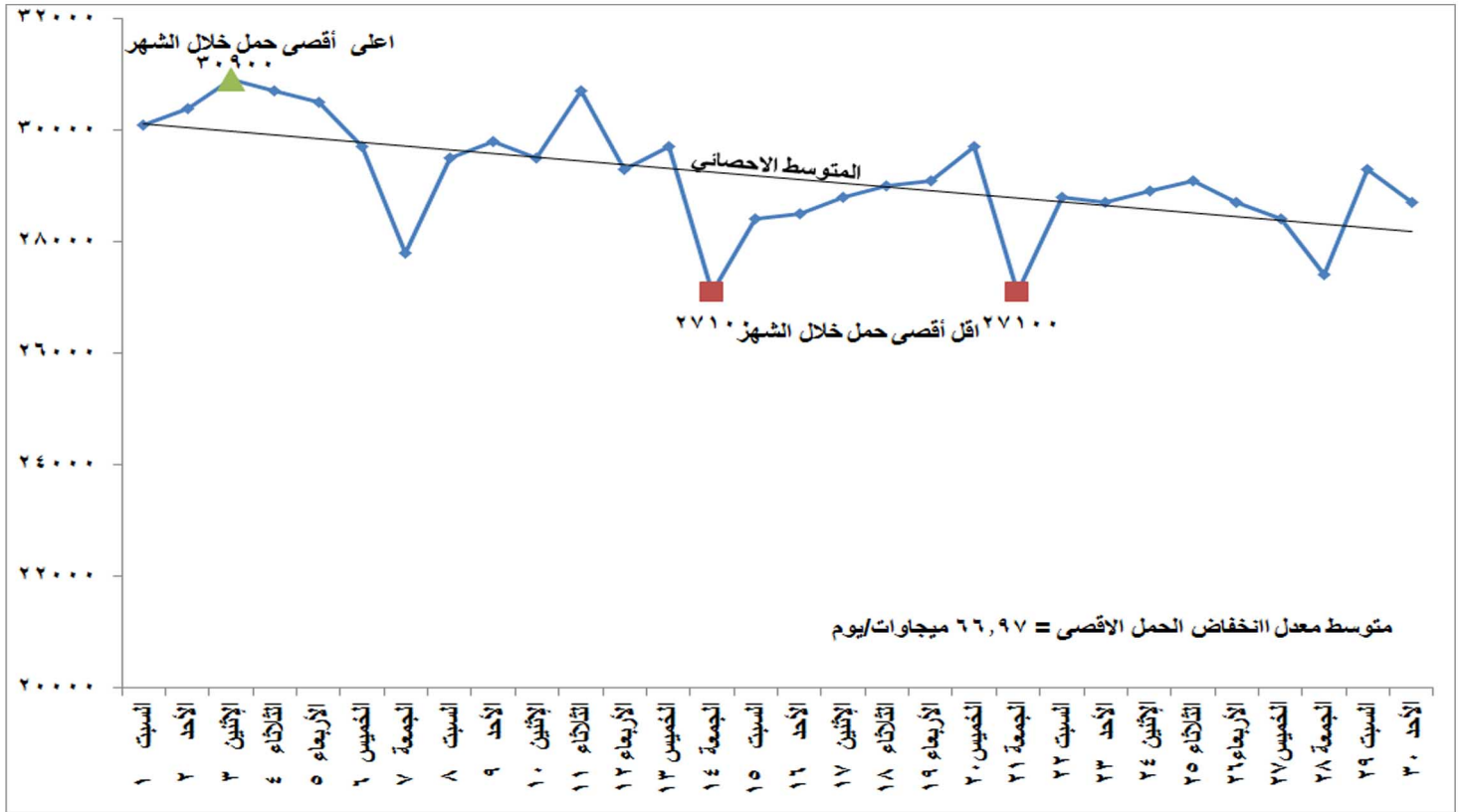
شكل (١) تطور الحمل الاقصى اليومي خلال شهر أكتوبر ٢٠١٨
