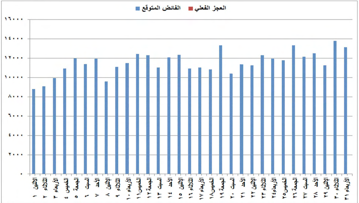
شكل (٧) الفائض والعجز المتوقع للقدرات خلال شهر أكتوبر ٢٠١٨
