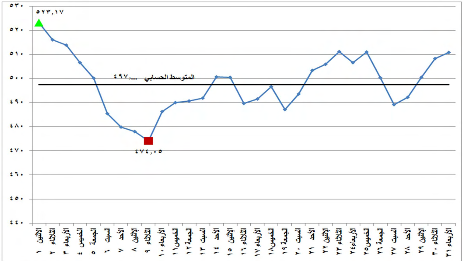
شكل (١٤) معامل انبعاثات غاز ثاني اكسيد الكربون المكافئ على مدى شهر أكتوبر ٢٠١٨
