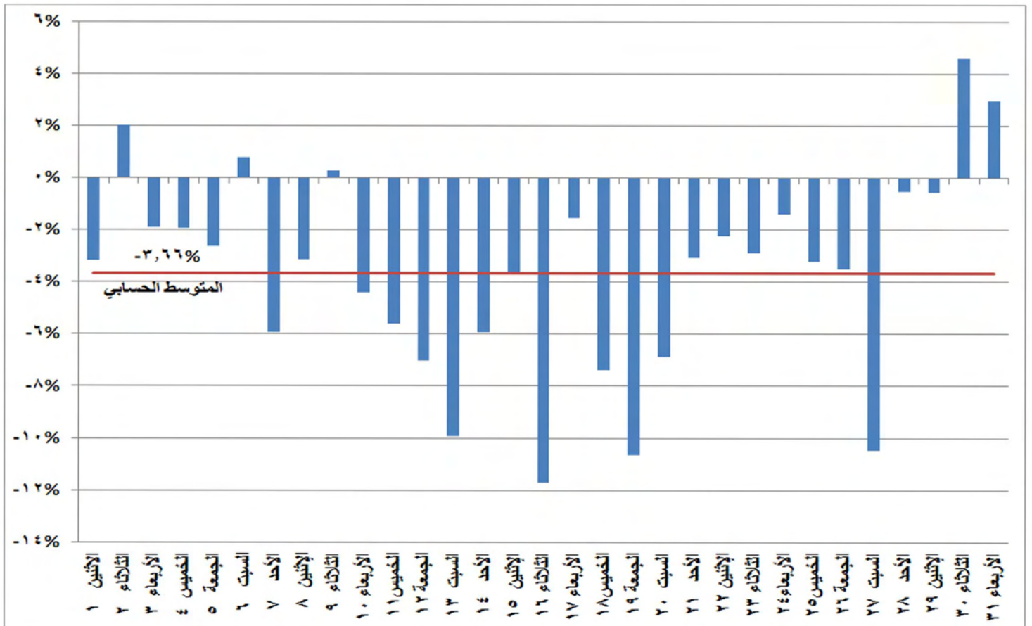
شكل (٢٤) نسب التغير في استخدام المصادر المائية في إنتاج الطاقة الكهربائية خلال شهر أكتوبر ٢٠١٨ مقارنة بالشهر المماثل من العام السابق
