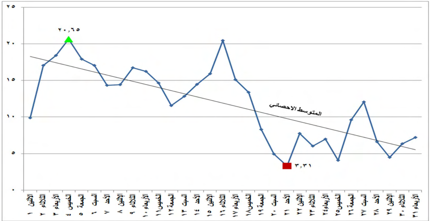
شكل (٢٥) الطاقة الكهربائية المنتجة من الرياح والشمس خلال شهر أكتوبر ٢٠١٨
