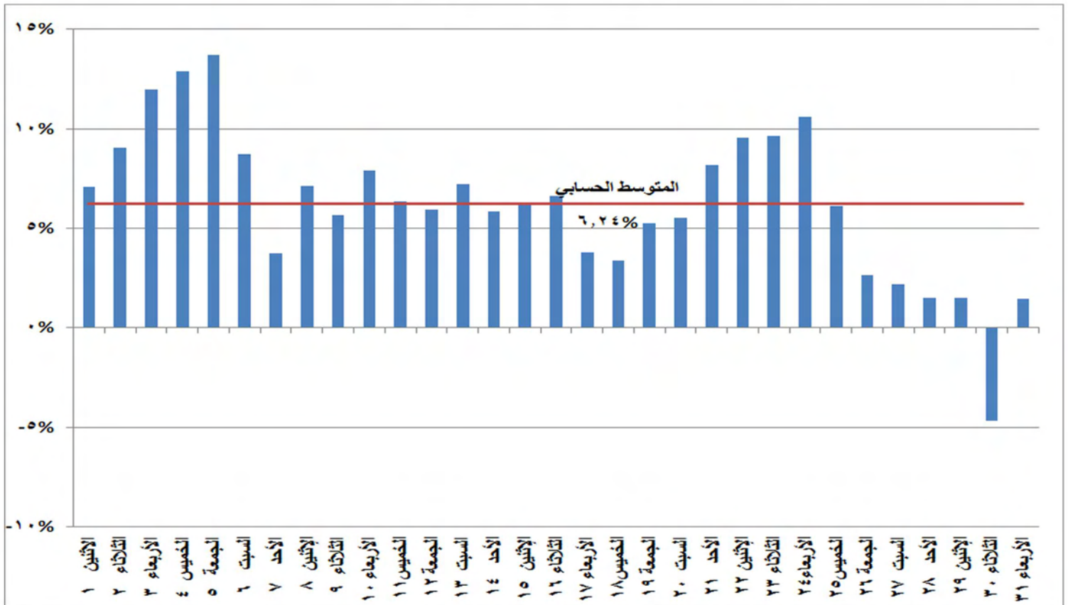
شكل (١٦) نسب التغير في الطاقة الكهربائية المنتجة خلال شهر أكتوبر ٢٠١٨ مقارنة بالشهر المماثل من العام السابق
