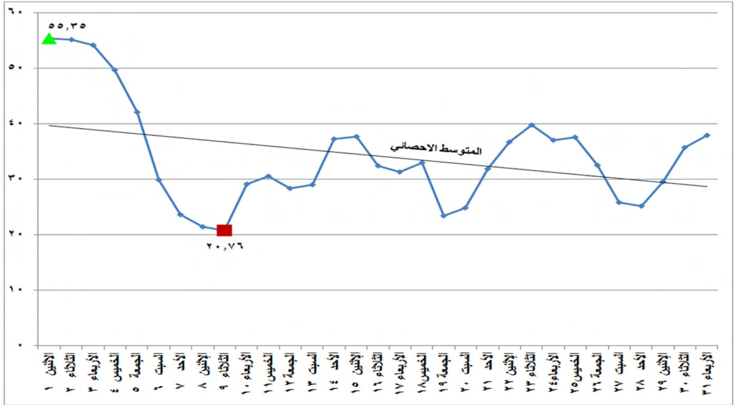
شكل (١٩) الطاقة الكهربائية المنتجة من المازوت خلال شهر أكتوبر ٢٠١٨
