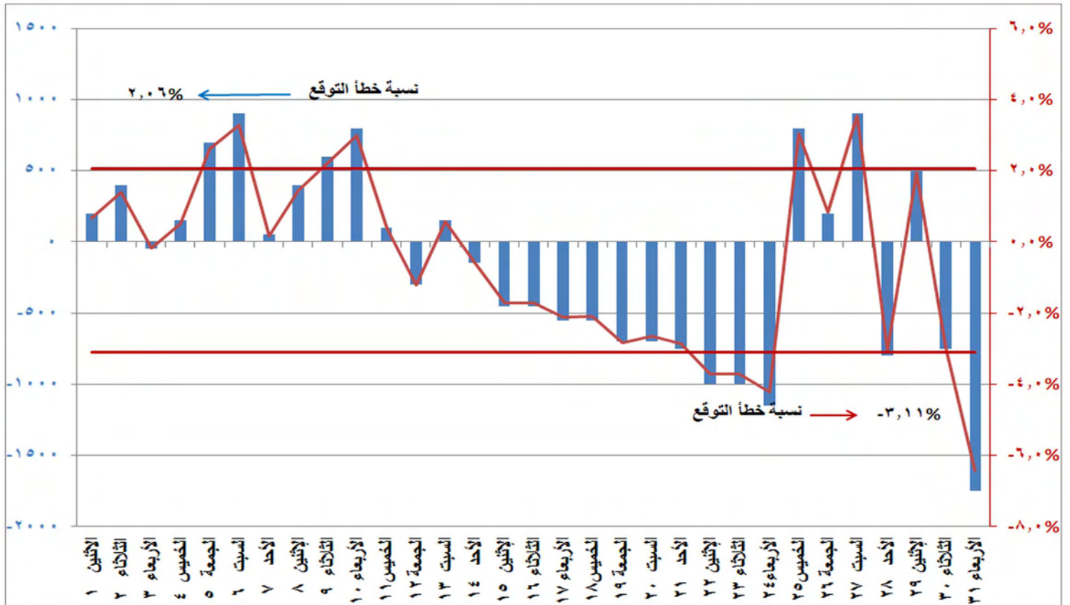
شكل (١٠) الفرق بين الحمل الأقصى المتوقع والمسجل فعليا ونسبة الفرق إلى الحمل المسجل فعليا خلال شهر أكتوبر ٢٠١٨
